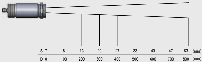
15:1 optics
